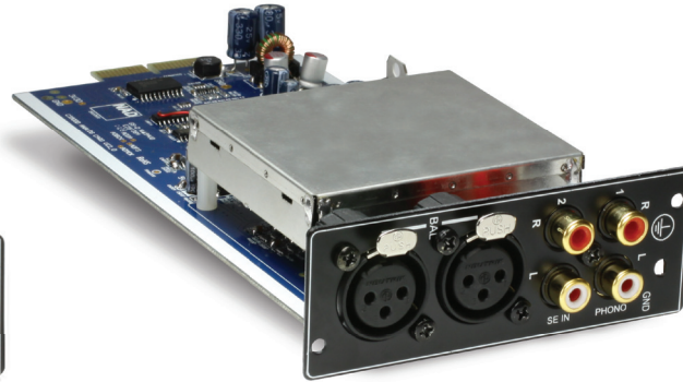
DD AP-1 Analogue Phono Module
