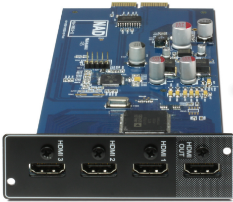
DD HDM-1 HDMI Module
